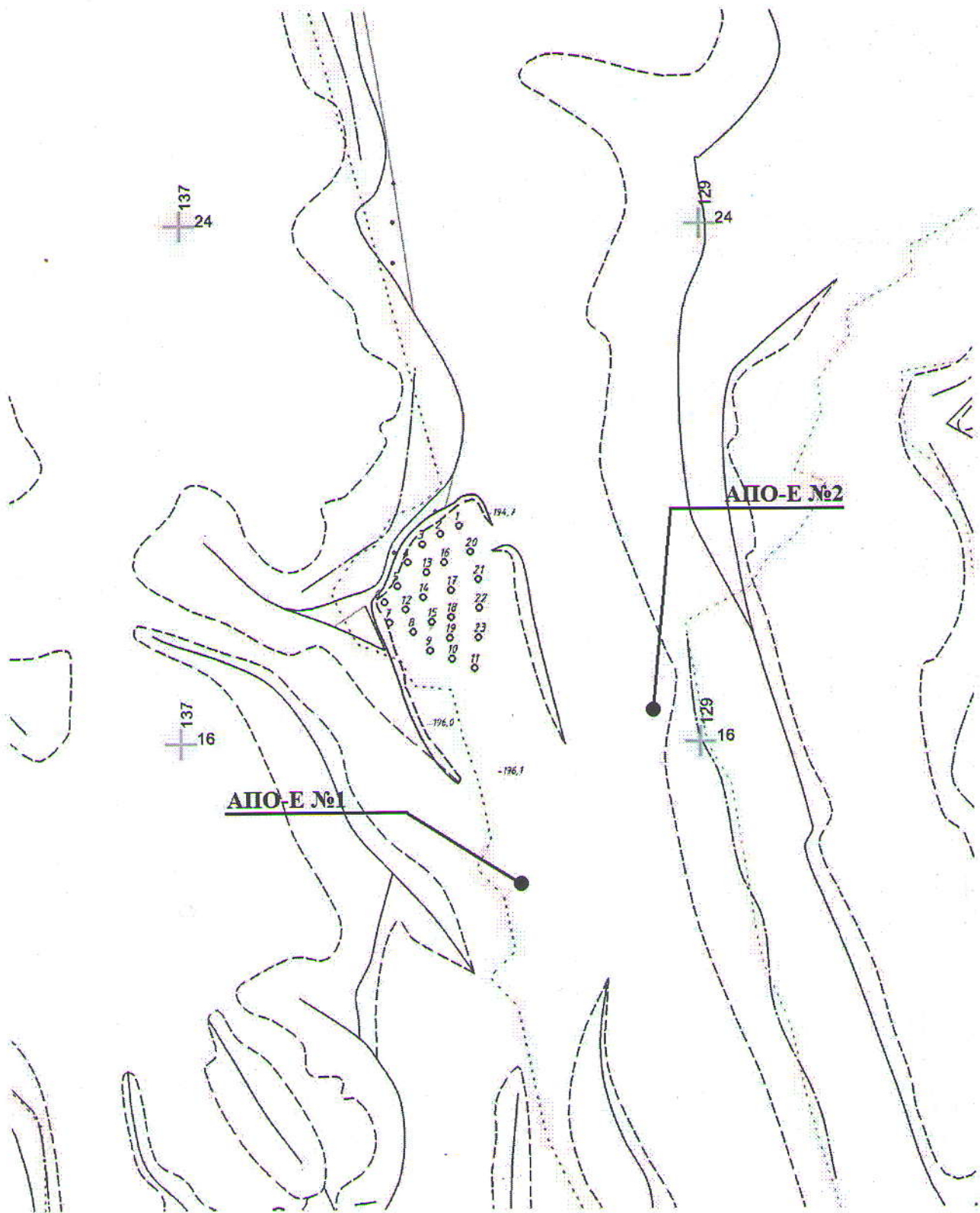
Рисунок 1 – Схема дослідного блоку (бл. №36 гор. -210 м від 19.10.2023 р.)
